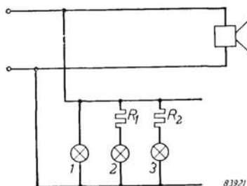
Fig. 99. Circuito per le misure della tensione d'uscita:
