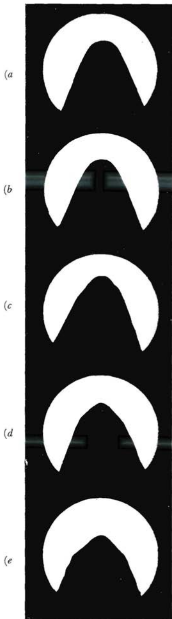
Fig. 40. Puntina di zaffiro per microscolto: nuova e dopo 75, 125, 175 e 225 ore.
