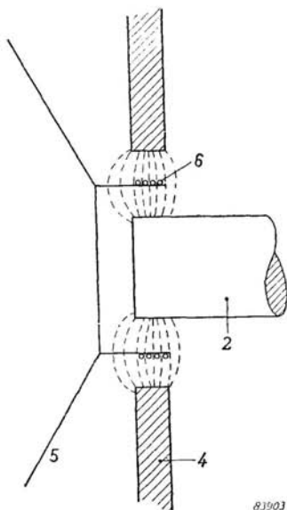
Fig. 70. Campo magnetico nel traferro di un altoparlante elettrodinamico: 2) Nucleo, 4) Piastra polare, 5) Cono, 6) Bobina mobile.
