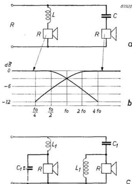
Fig. 97. Filtro di divisione: a) Schema per un'attenuazione di 6 dB per ottava, b) Caratteristica di frequenza dello schema a), c) Schema per un'attenuazione di 12 dB per ottava.
