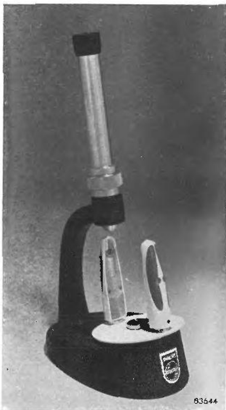
Fig. 43. Microscopio per il controllo delle puntine.
