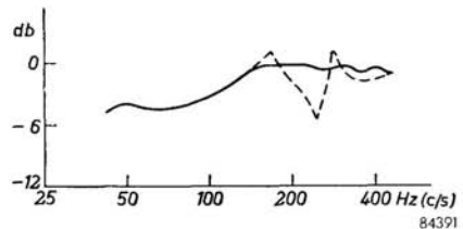
Fig. 49. Influenza del braccio del pick-up nella riproduzione dei bassi.
