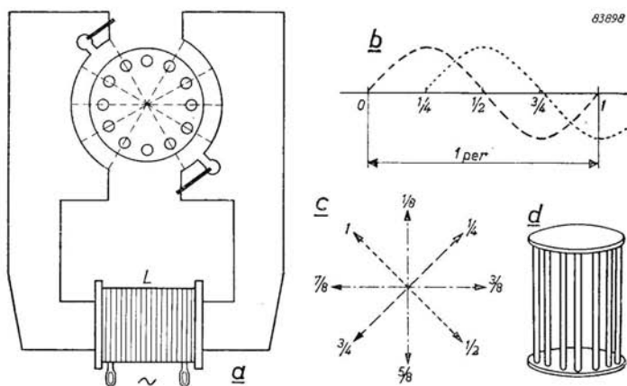
Fig. 44. Principio di funzionamento del motore gramofonico a due poli.
