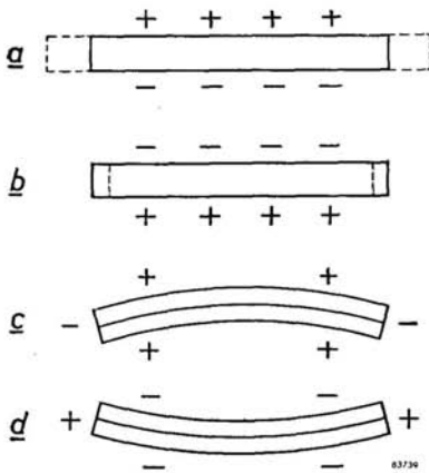
Fig. 17. Principio di funzionamento del pick-up a cristallo.
