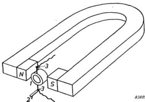
Fig. 22. Pick-up elettrodinamico.
