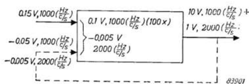
Fig. 64. Rappresentazione schematica della controreazione.
