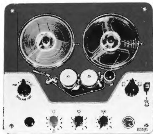
Fig. 108b. Registratore magnetico non professionale; da sinistra a destra: testina di cancellazione, testina di registrazione e di riproduzione.
