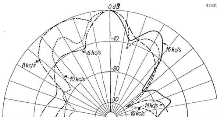
Fig. 80. Diagramma d'irradiazione: a) Altoparlante tipo 9770. b) Altoparlante tipo 9770 M.
