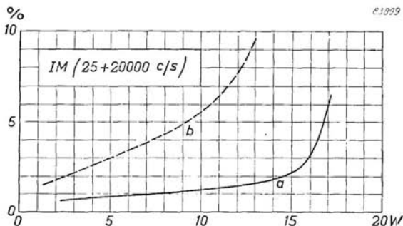
Fig. 58. Curve d'intermodulazione: a) amplificatore tipo AG 9000 b) amplificatore normale.
