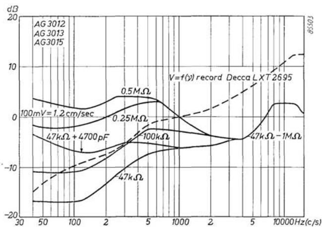
Fig. 117. Caratteristiche di riproduzione dei pick-up a cristallo tipi AG 3012, AG 3013 ed AG 3015 rilevate col disco Decca LXT 2695 (33 \frac{1}{3} giri/minuto).
