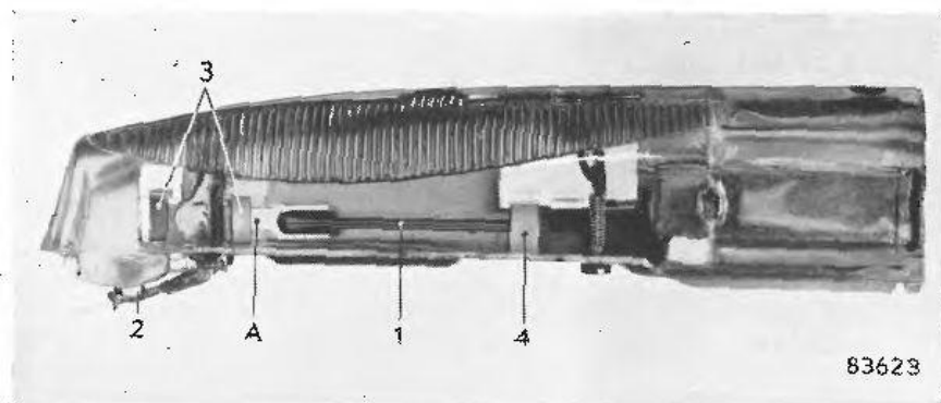
Fig. 18. Pick-up a cristallo tipo AG 3010.
