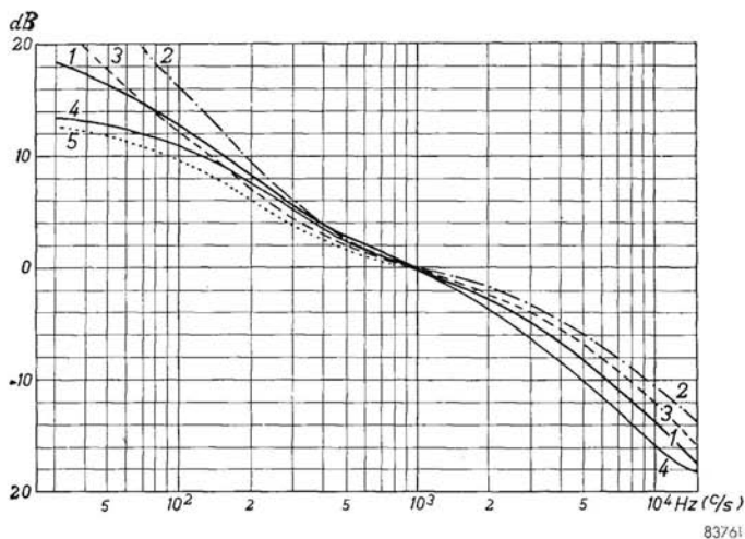
Fig. 37. Le principali caratteristiche di riproduzione Vedi anche la tabella dopo la fig. 38.
