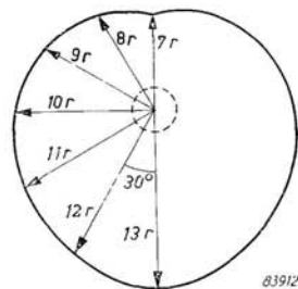
Fig. 87. Schermo acustico a forma di cuore. 7r = a in fig. 85.
