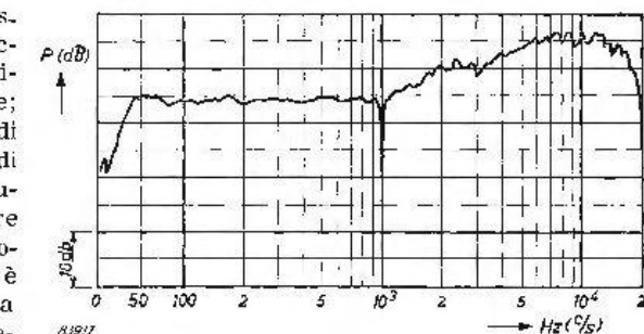
Fig. 91. Curva della pressione sonora della combinazione di altoparlanti tipo AD 5002 (acoustic box con proiettori).
